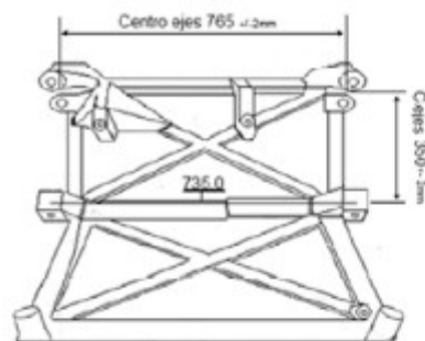
Dibujo subchasis con medidas
