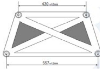
Dibujo refuerzo suspensión delantera
