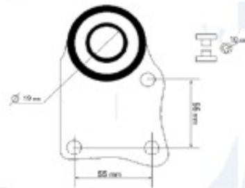
Dibujo y medidas rótula inferior
