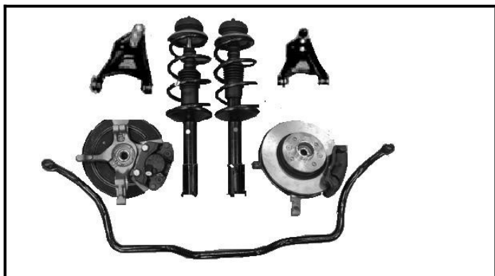
Suspensión delantera completa desmontada
