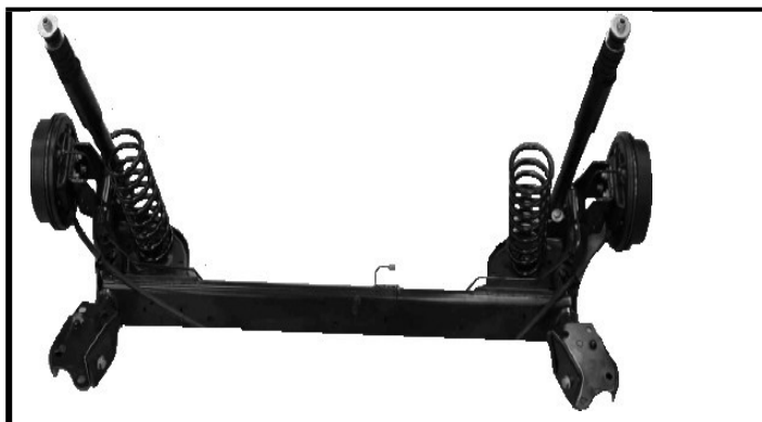
Suspensión trasera completa desmontada
